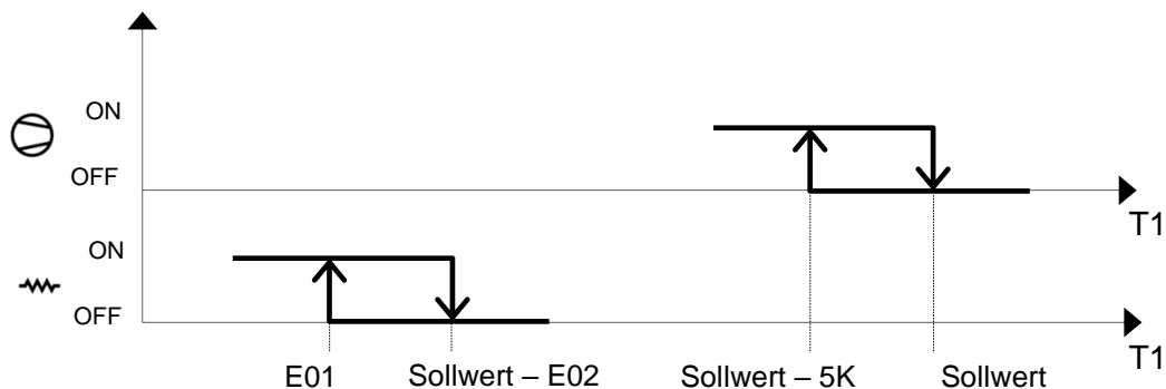
Abbildung 10: Schaltdiagramm besondere Betriebsweise E-Heizstab
