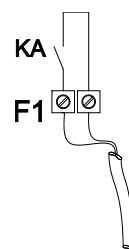
Abbildung 3: Schalteingang F1
