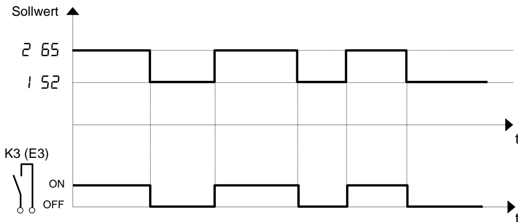
Abbildung 12: Schaltdiagramm Sollwerterhöhung
