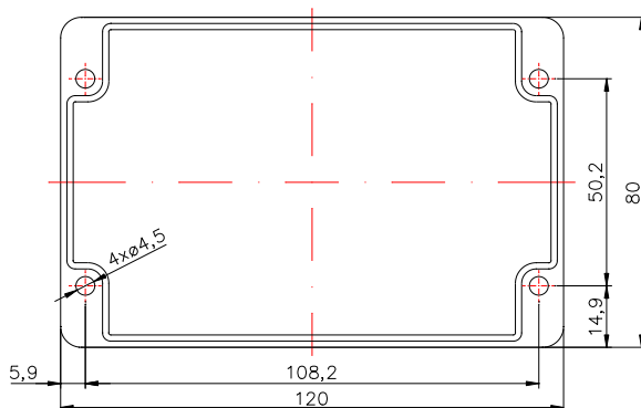
Abbildung 2: Bohrschablone
