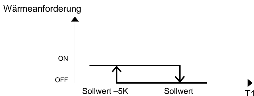
Abbildung 6: Diagramm Wärmeanforderung
