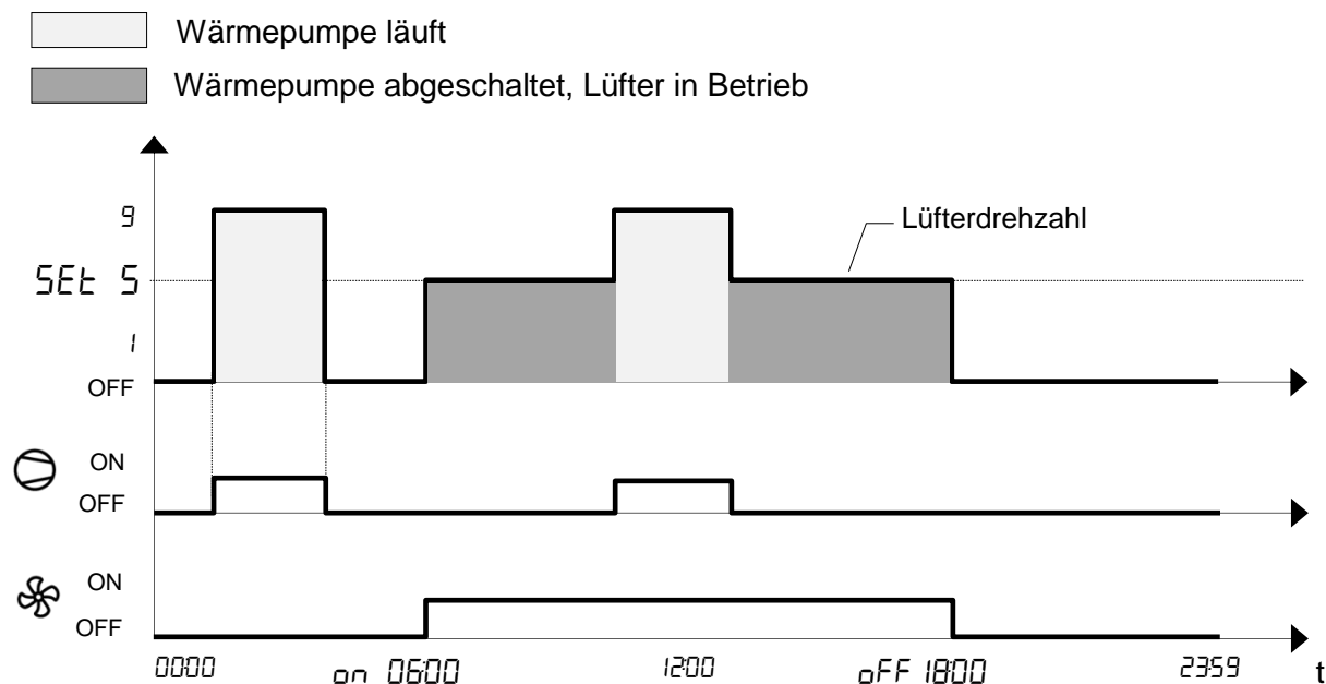
Abbildung 8: Diagramm Lüftungsbetrieb - Wärmepumpenbetrieb
