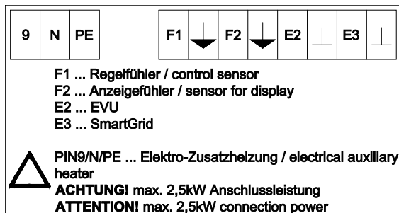
Abbildung 1: Anschlussplan
