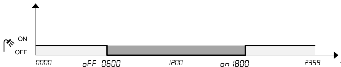
Abbildung 7: Diagramm Warmwasser Zeitprogramm
