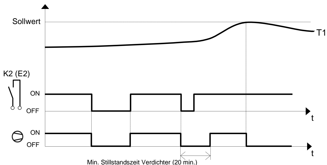
Abbildung 11: Schaltprogramm externe Abschaltung
