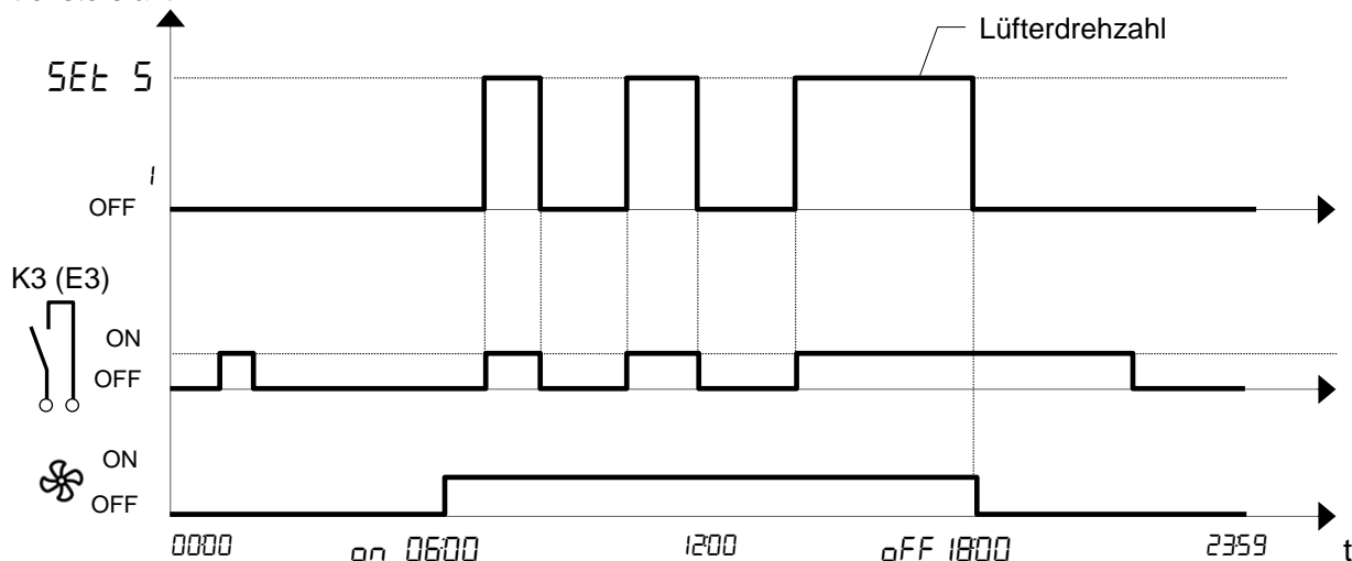
Abbildung 9: Diagramm Lüftung extern gesteuert (Par. A04 = 3)
