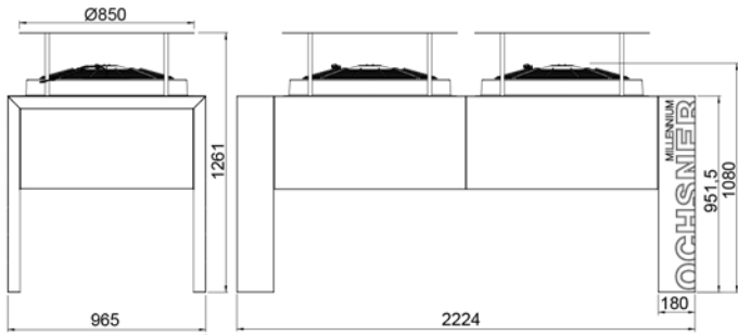
SPLIT-VERDAMPFER VHS-M 80
